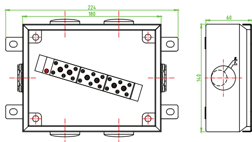
1. Otwór pod dławik M32 2. Otwór pod dławik M20
