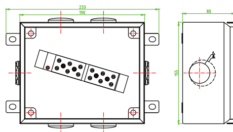
1. Otwór pod dławik M32 2. Otwór pod dławik M40
