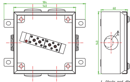
1. Otwór pod dławik M32 2. Otwór pod dławik M20
