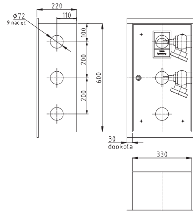
Wymiary szafki (wnęki)
