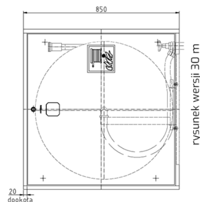
Wymiary hydrantu
