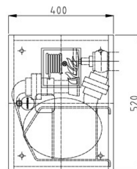
Wymiary hydrantu
