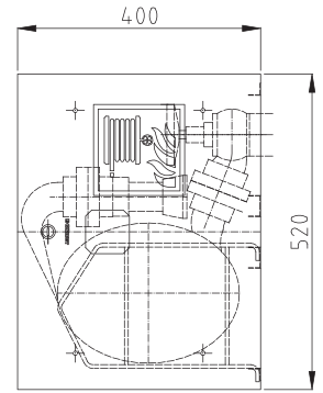
Wymiary hydrantu
