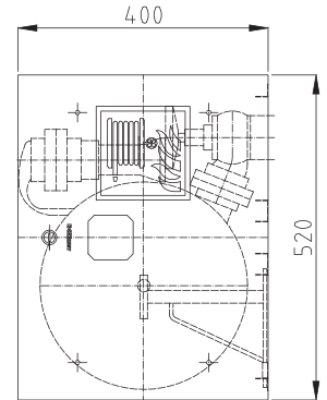
Wymiary hydrantu
