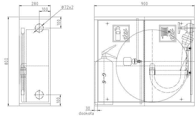
Wymiary hydrantu
