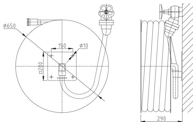
Wymiary hydrantu
