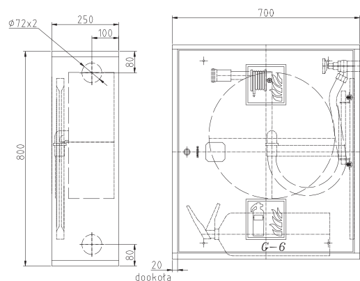
Wymiary hydrantu
